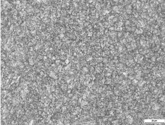
熱処理後のミクロ組織、倍率500倍。
