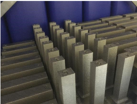
AM Dievarと1.2709(マルエージング鋼)およびAM H13(SKD61)の比較。垂直方向に造形し、硬さ 46~48 HRC に熱処理。AM Dievarはミクロ組織が微細なため、優れた靱性値を示します。
