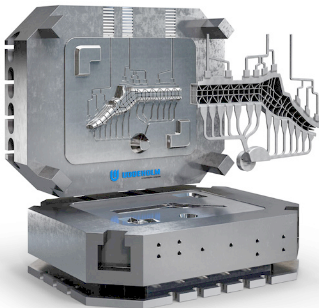
構造部品用のダイカスト金型の例
